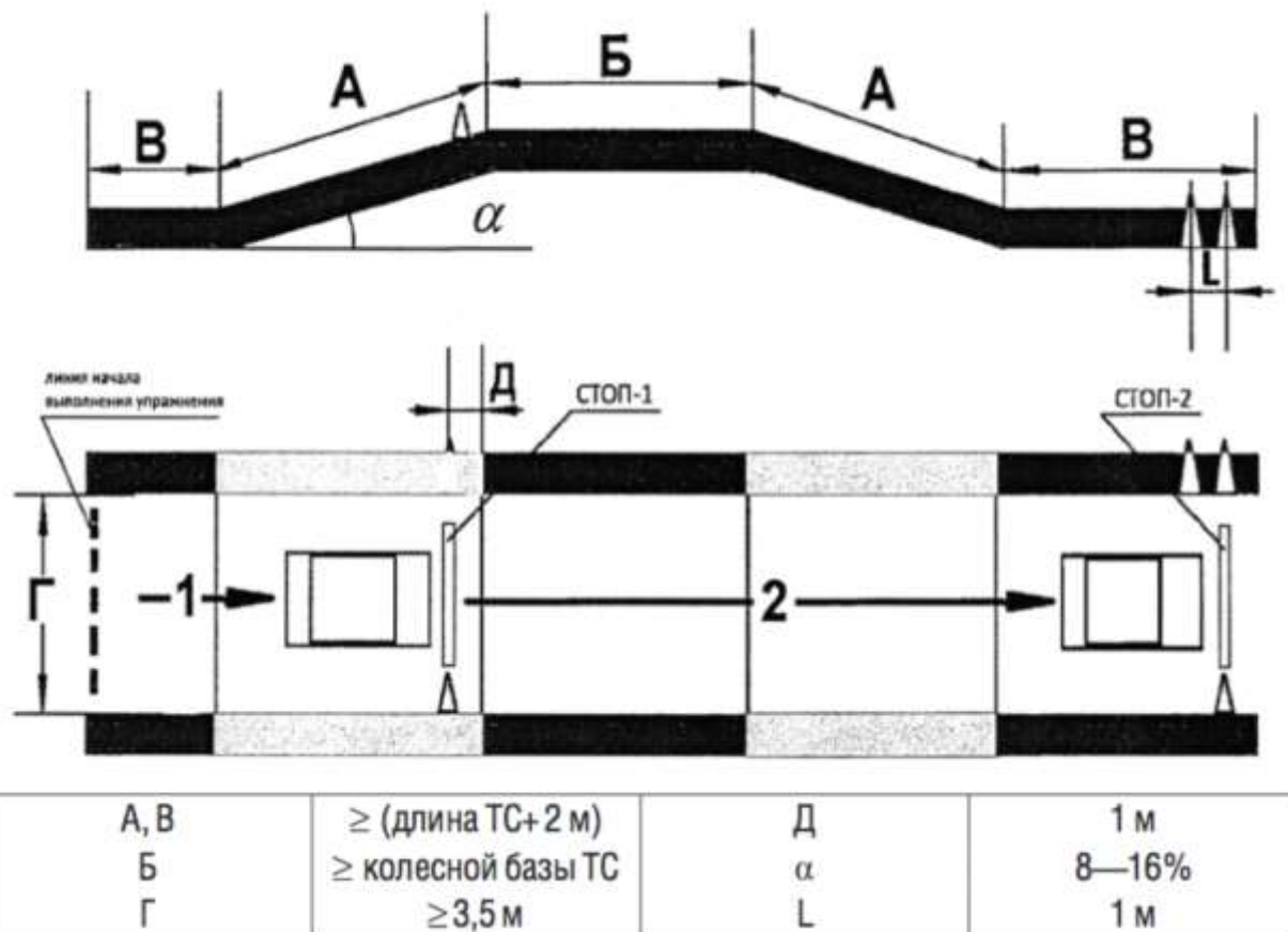
Рисунок 7. Схема и размеры упражнения N 4
