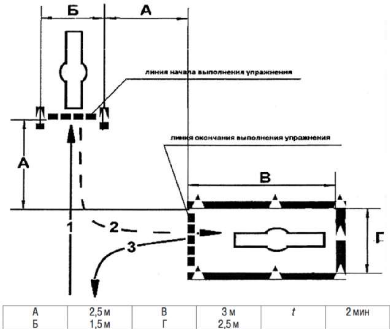
Рисунок 5. Схема и размеры упражнения N 2
