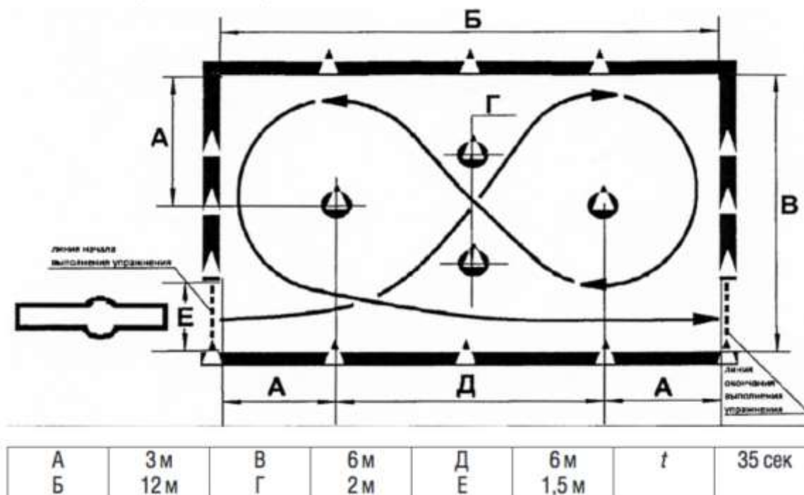
Рисунок 1. Схема и размеры элемента упражнения N 1 - "Габаритная восьмерка"
